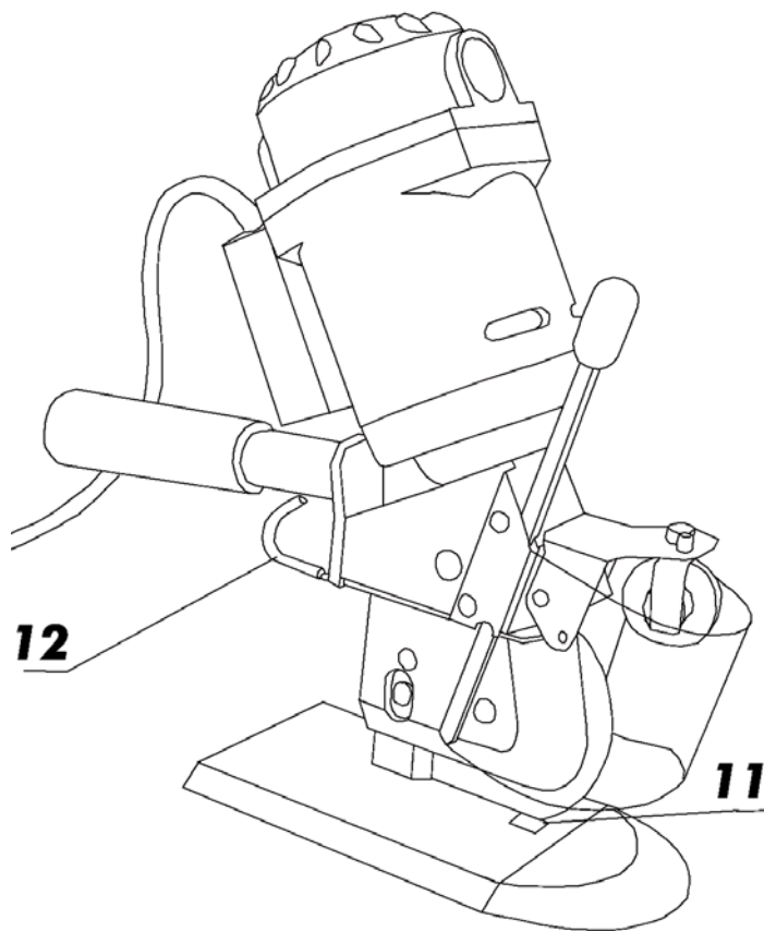
Рис. 1б. Общий вид раскройной машины (правая сторона)
