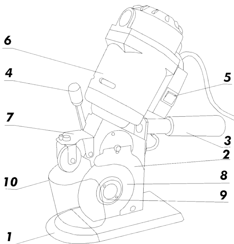
Рис. 1а. Общий вид раскройной машины (левая сторона)
